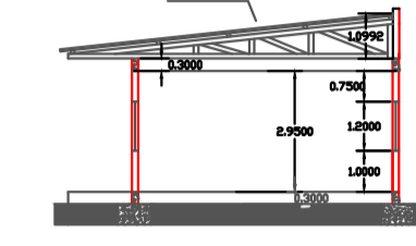
CORTE EF ESC 1:200
