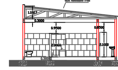
CORTE CD ESC 1:200
