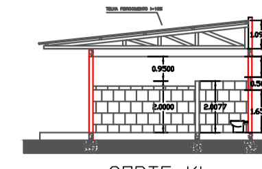
CORTE KL ESC 1:200
