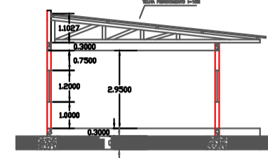
CORTE AB ESC 1:200
