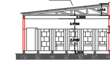
CORTE GH ESC 1:200
