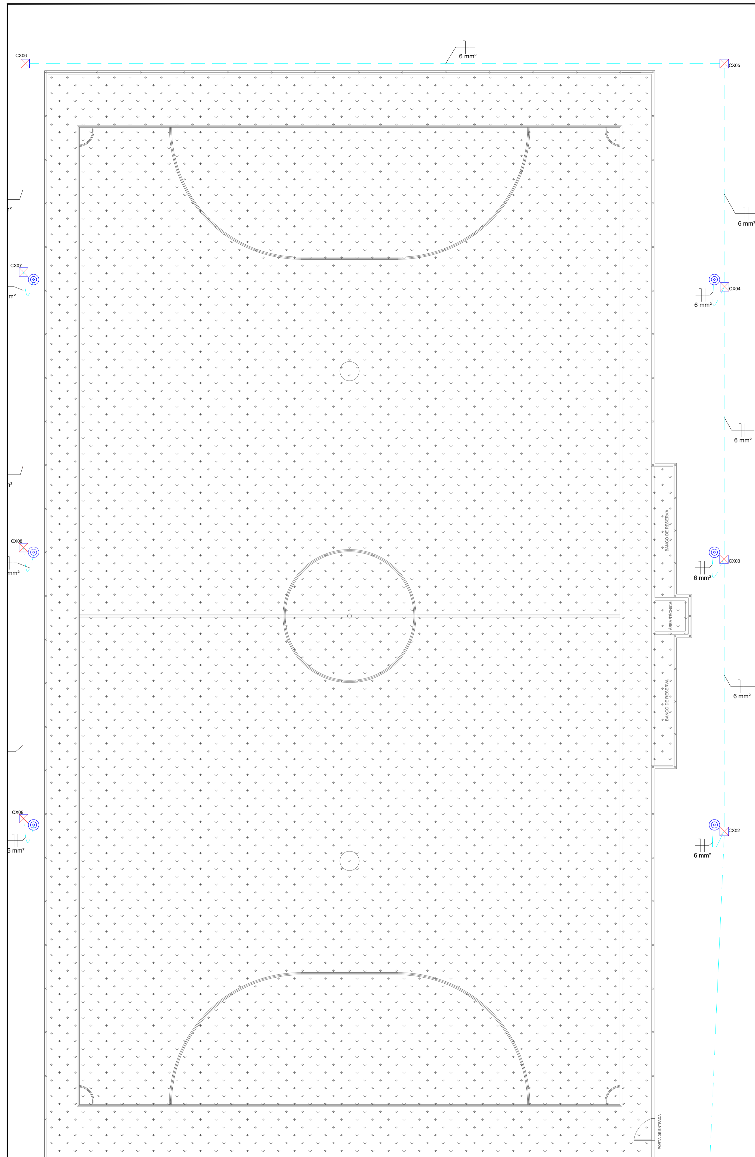
Planta de Distribuição Elétrica Esc: 1/100
