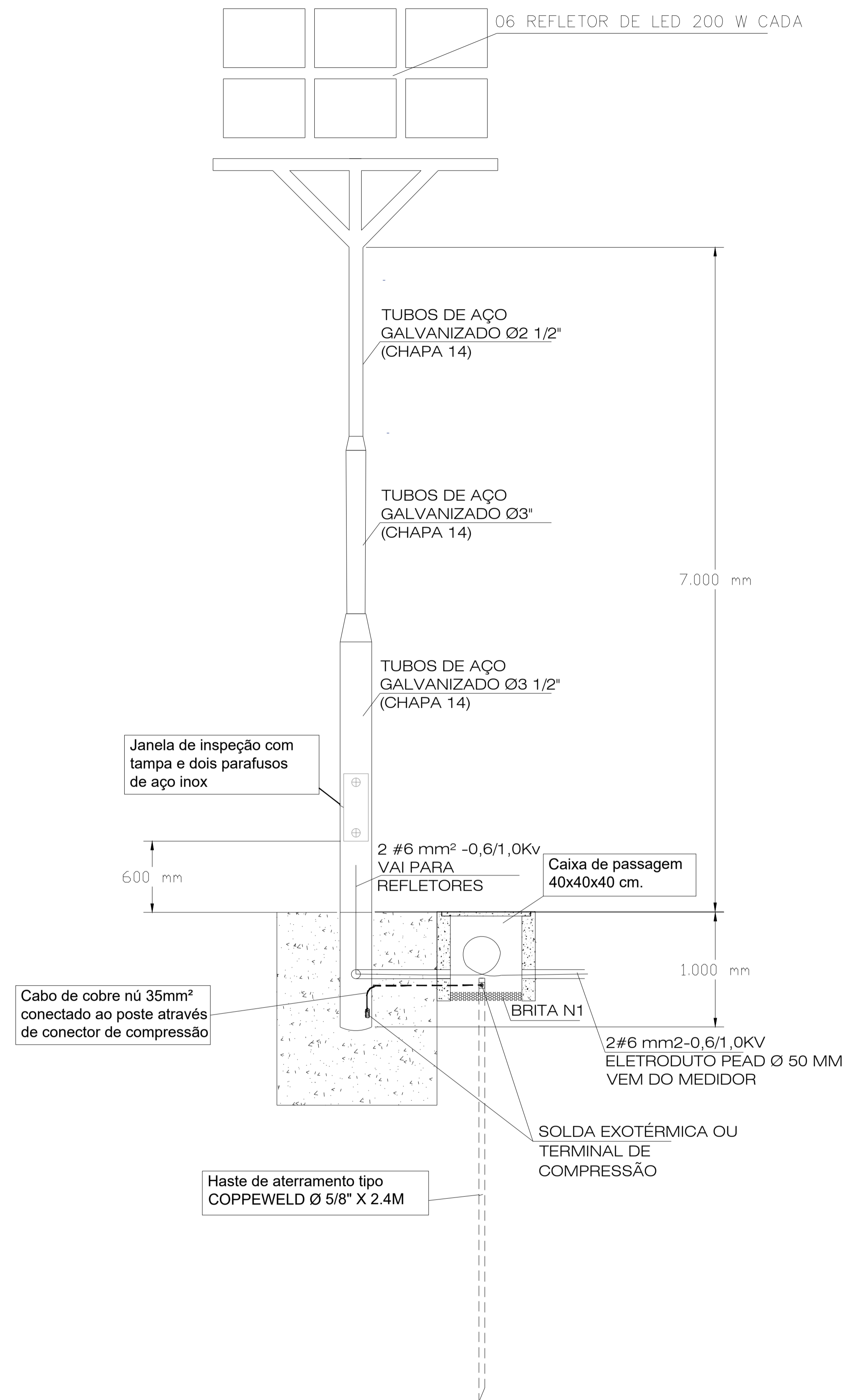
Detalhes construtivos - Postes com Refletores Esc: s/escala
