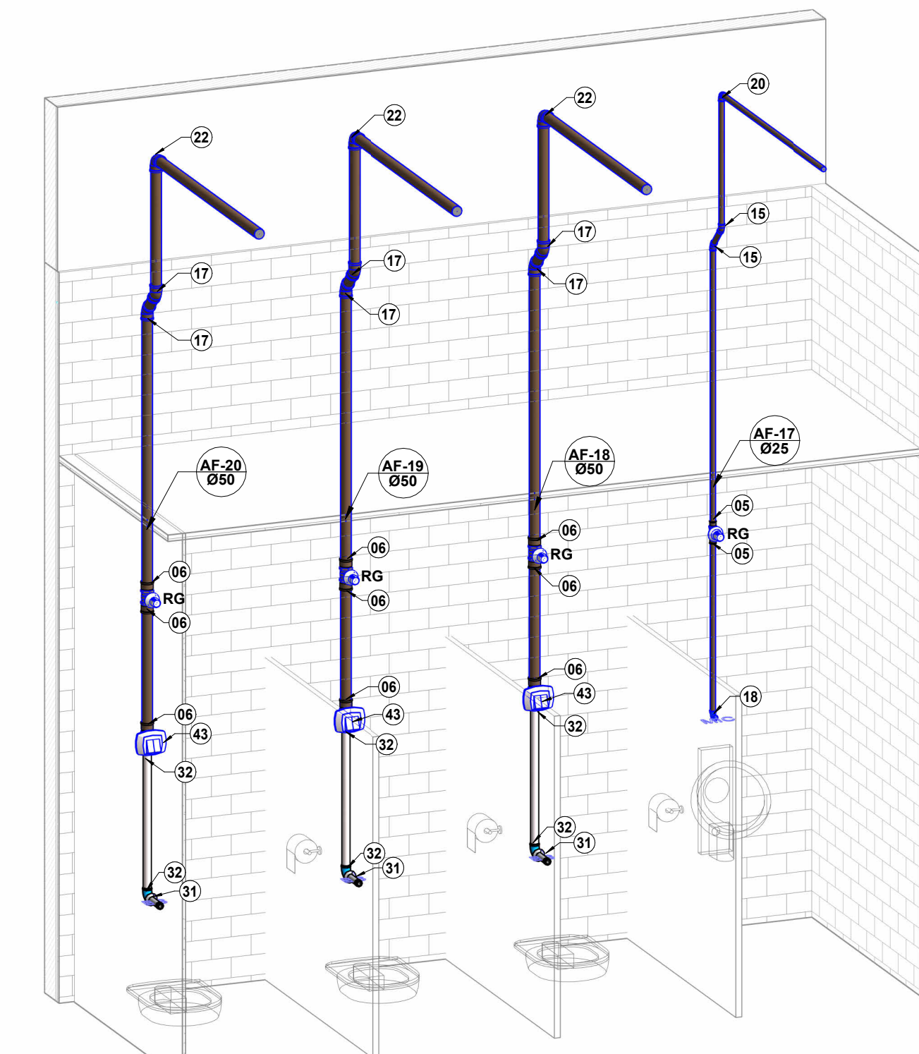
DET.H7
