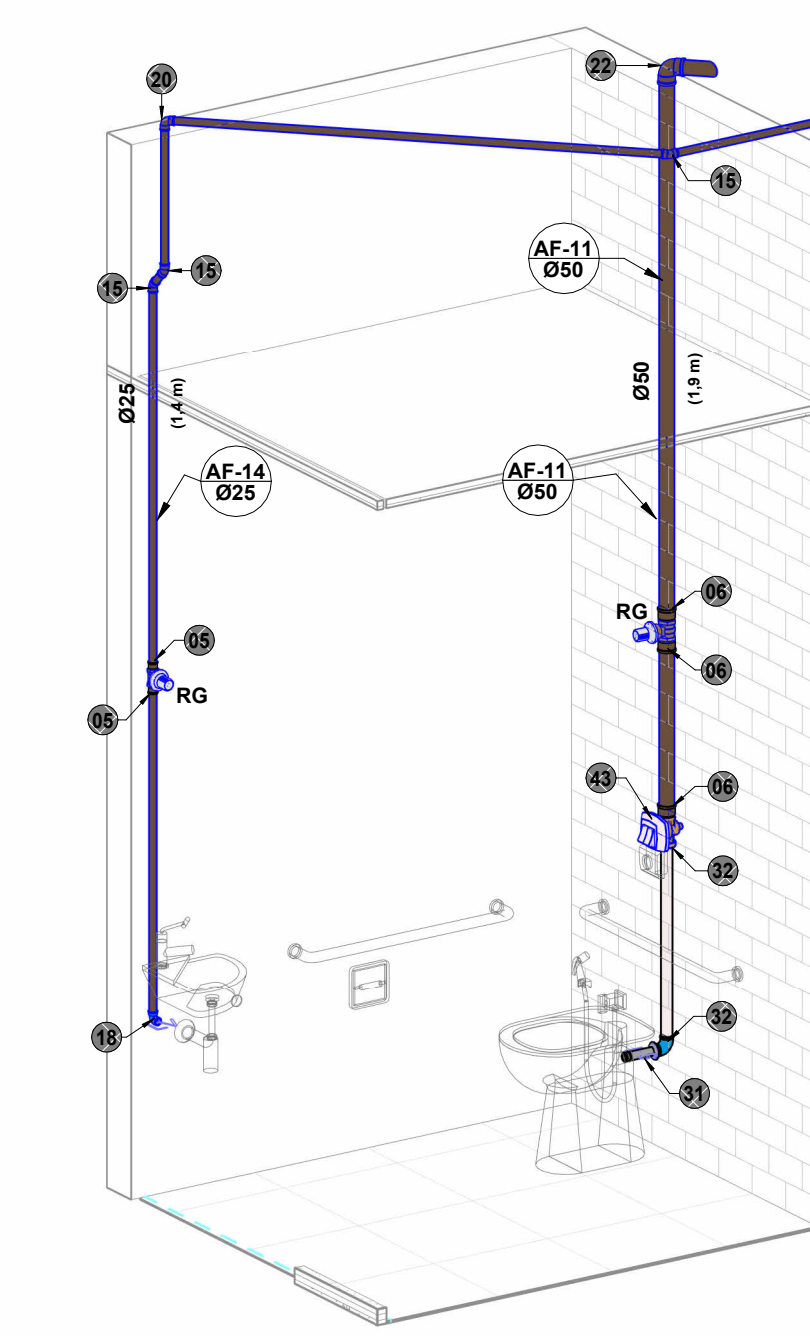
DET.H4
