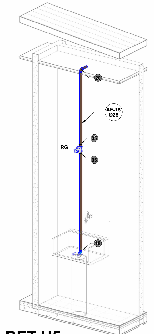
DET.H5
