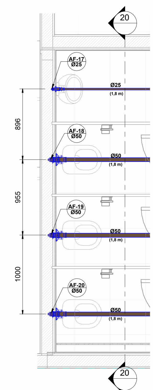
DET.H7 1 : 25
