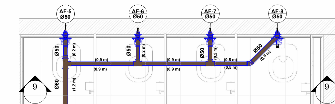
DET.H2 1 : 25
