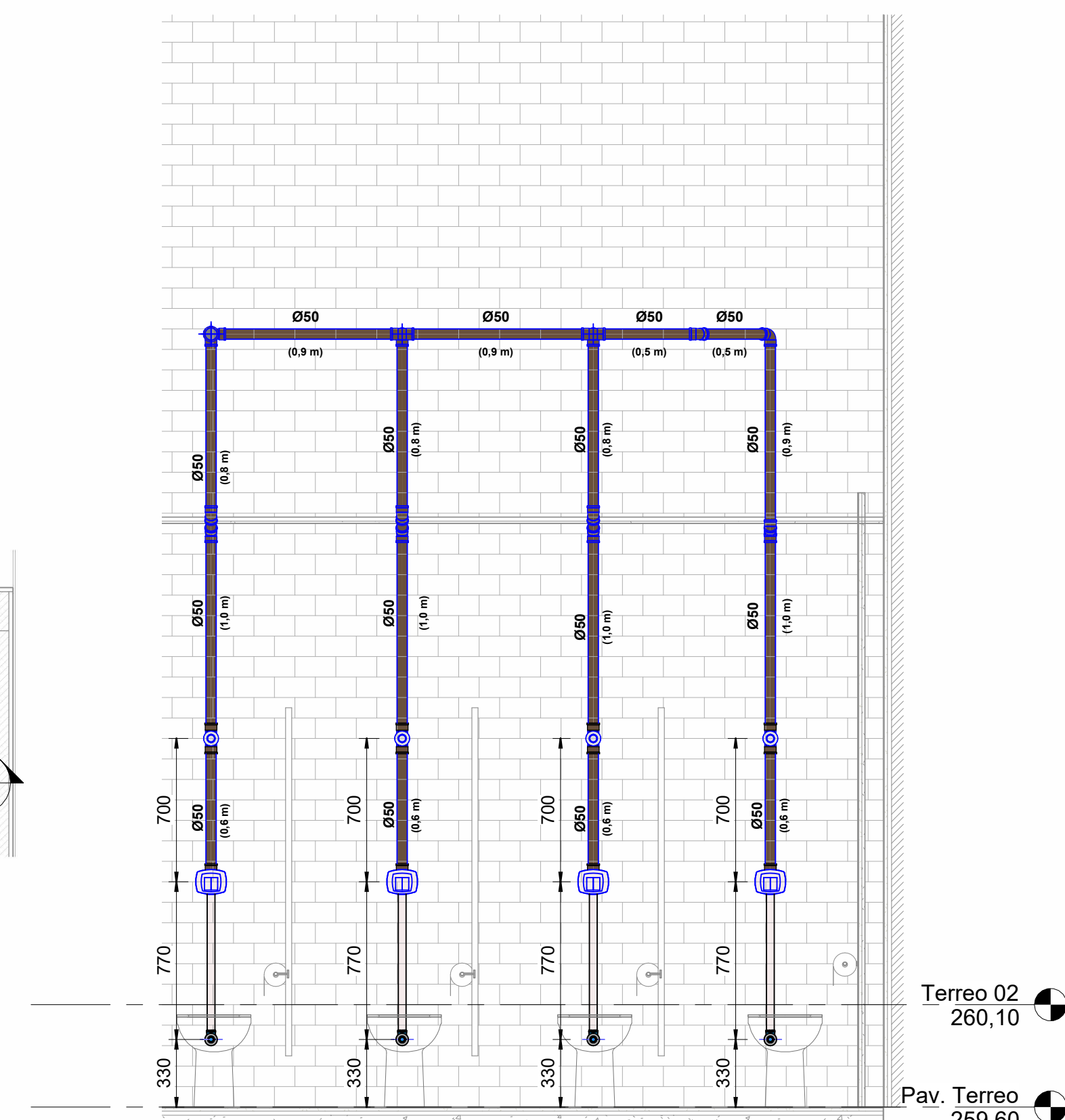
DET.H2 1 : 25
