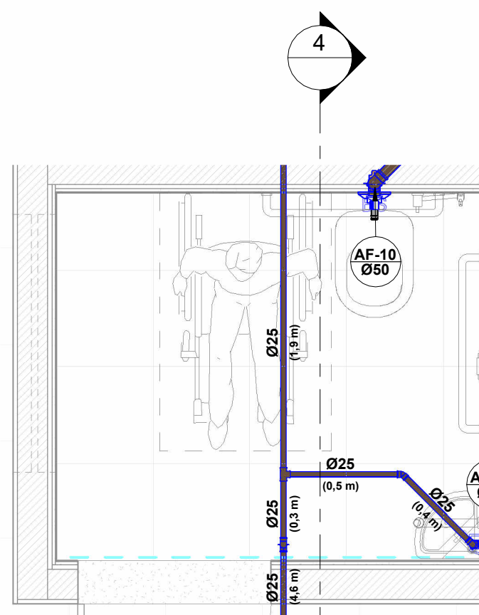
DET.H4 1 : 25
