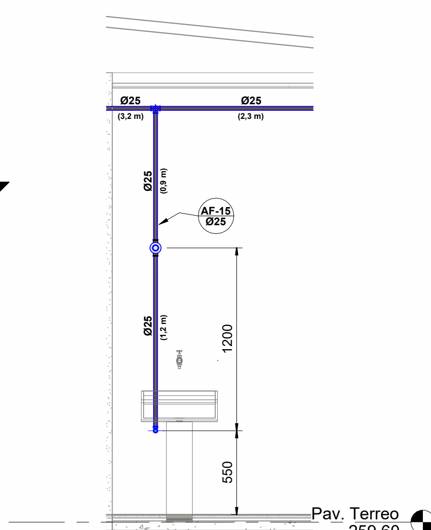
DET.H5 1 : 25
