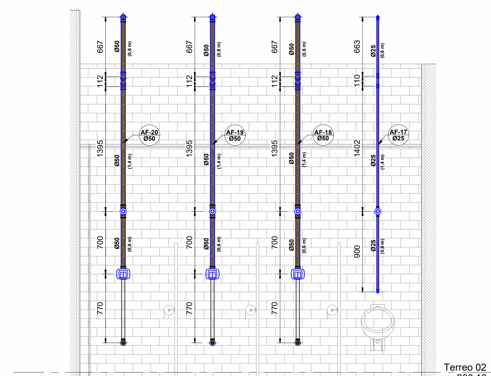
DET.H7 1 : 25
