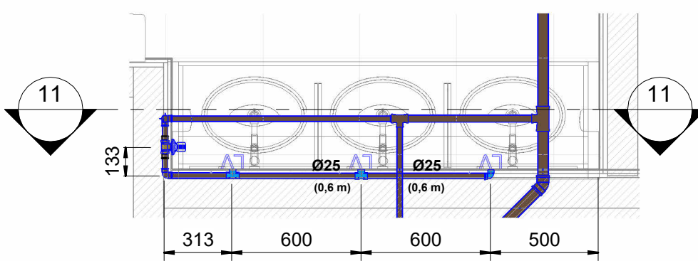
DET.H3 1 : 25
