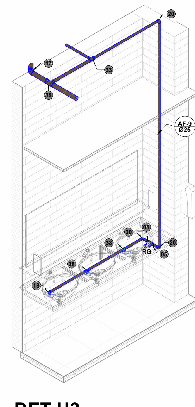
DET.H3
