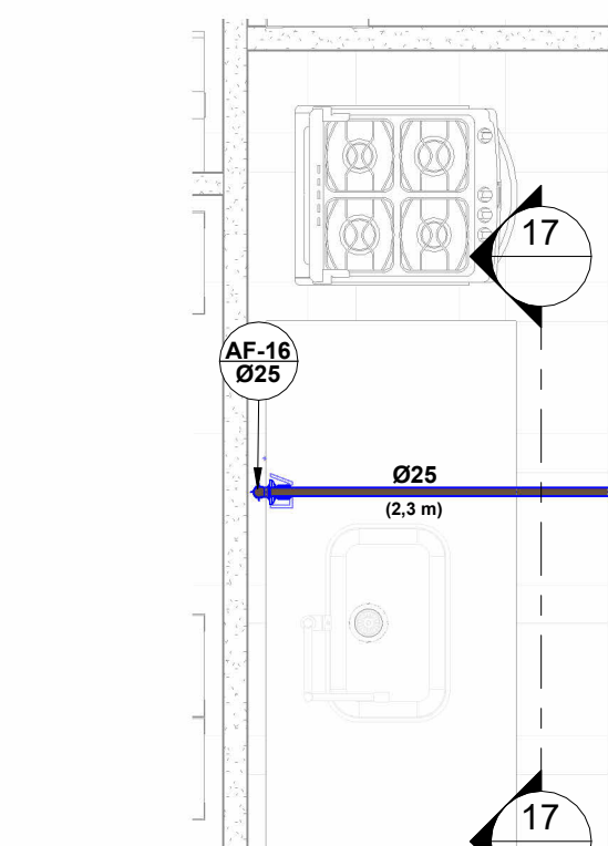
DET.H6 1 : 25
