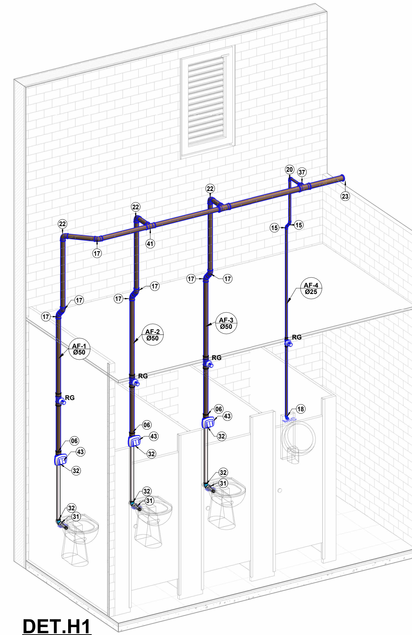
DET.H1
