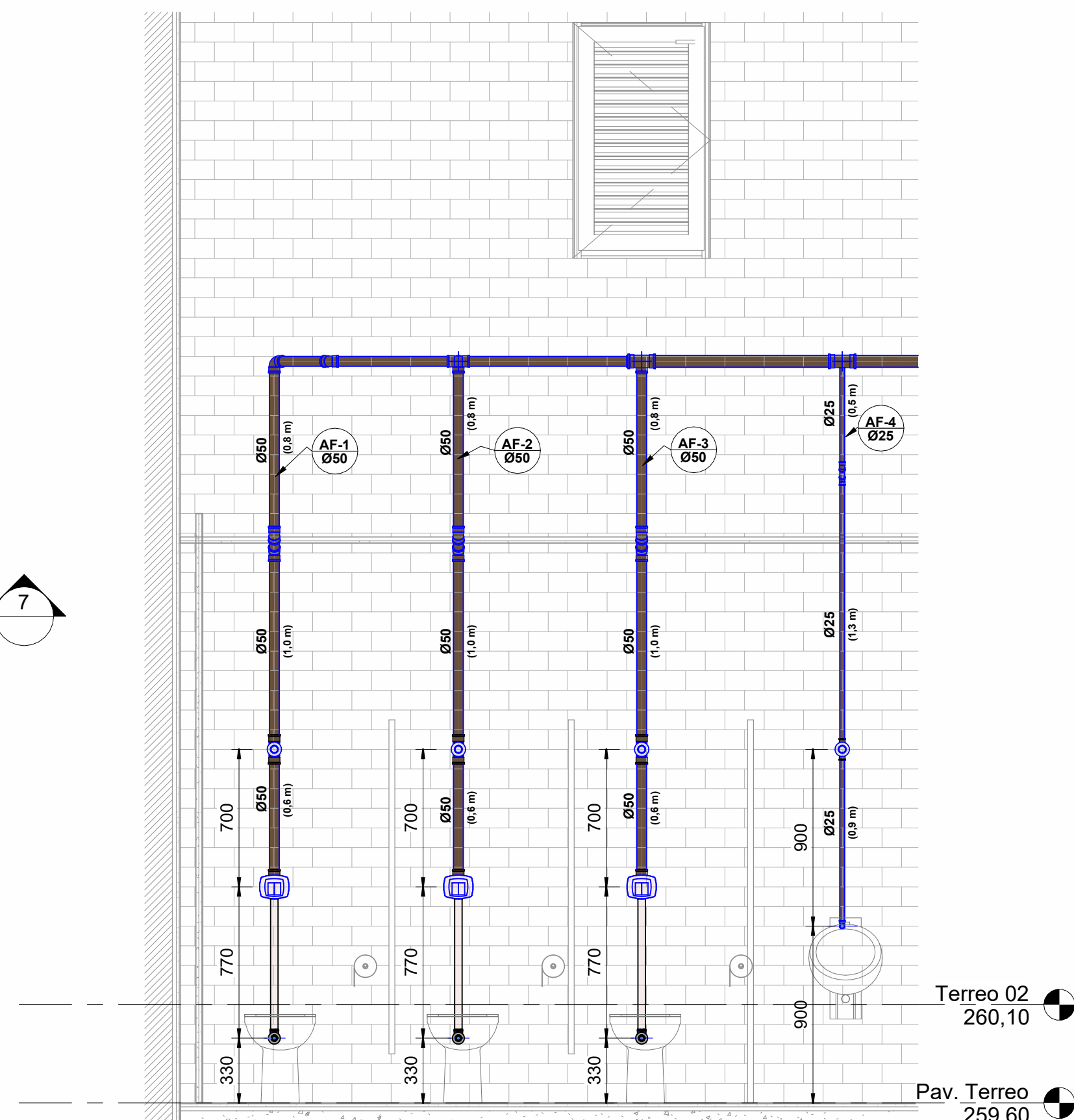
DET.H1 1 : 25
