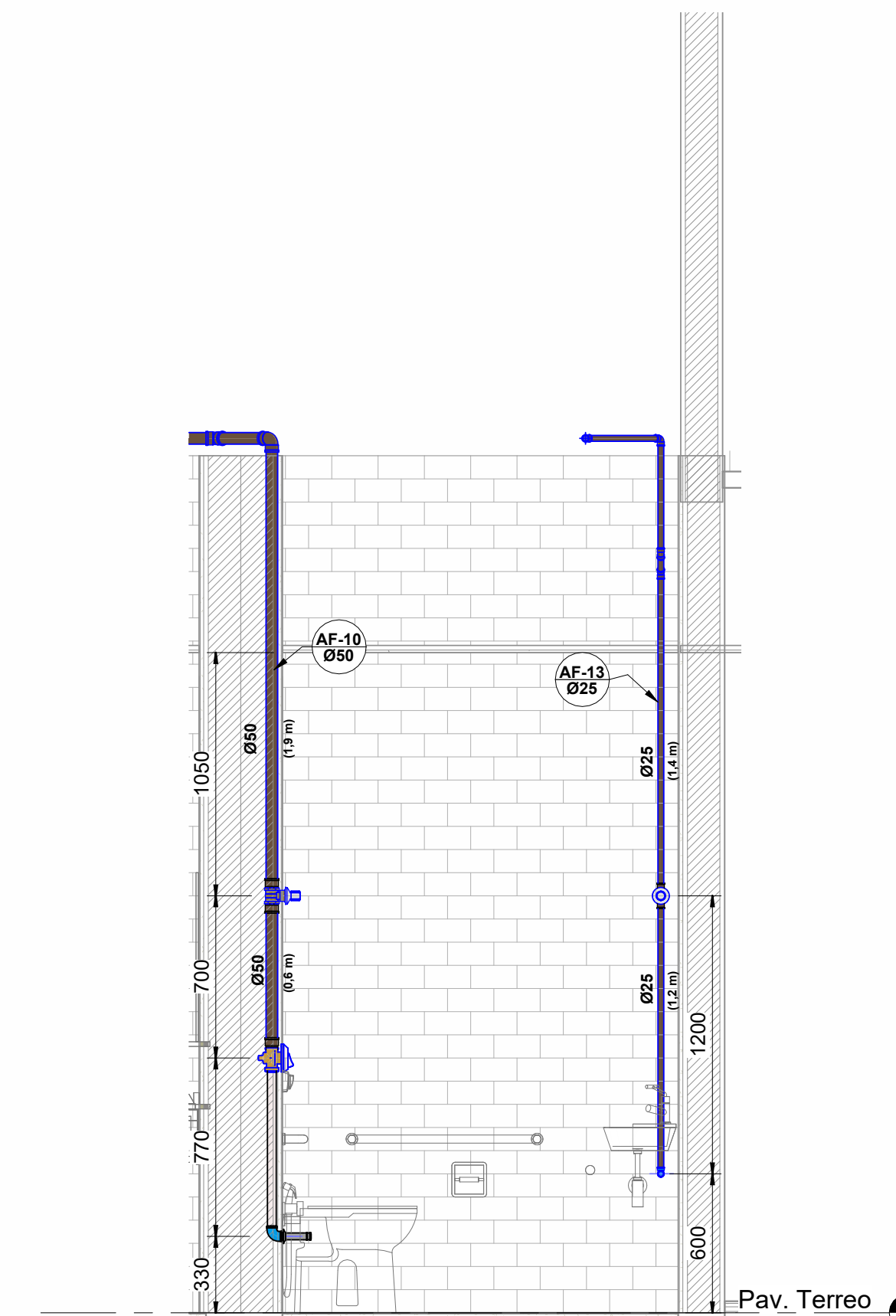
DET.H4 1 : 25
