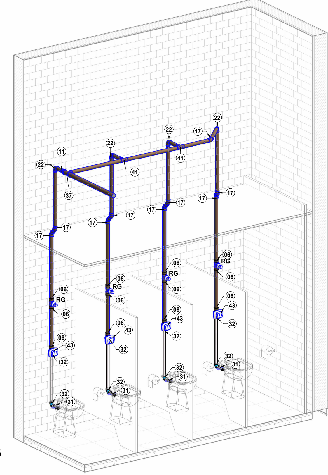
DET.H2
