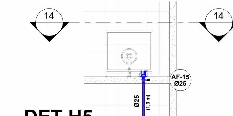
DET.H5 1 : 25
