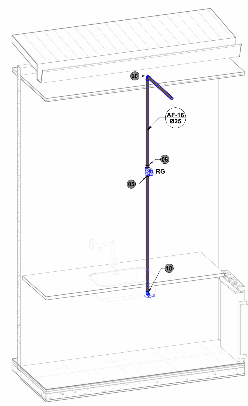
DET.H6
