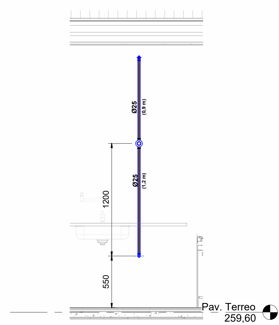
DET.H6 1 : 25
