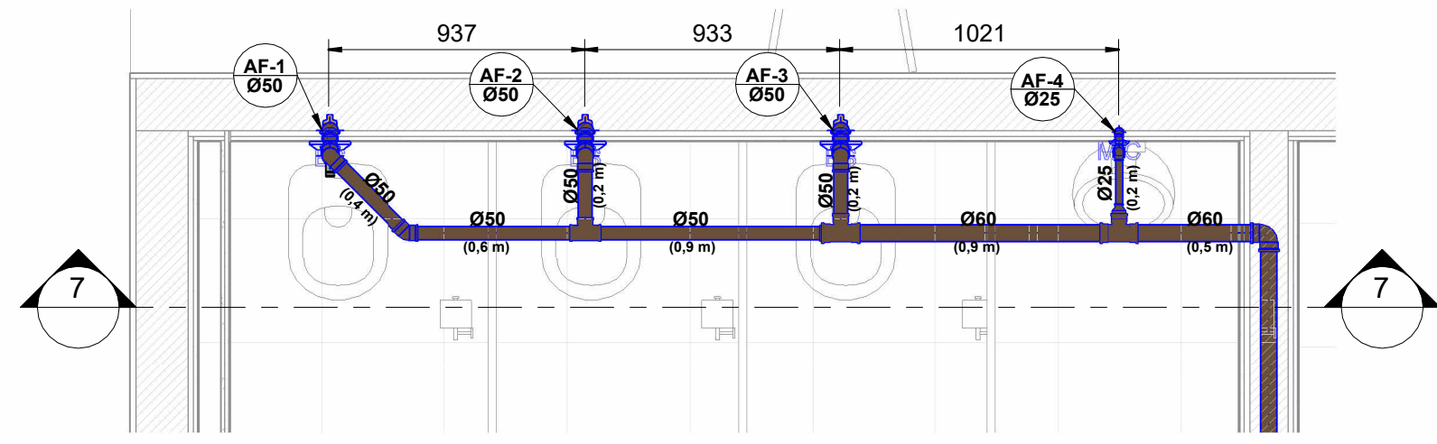
DET.H1 1 : 25
