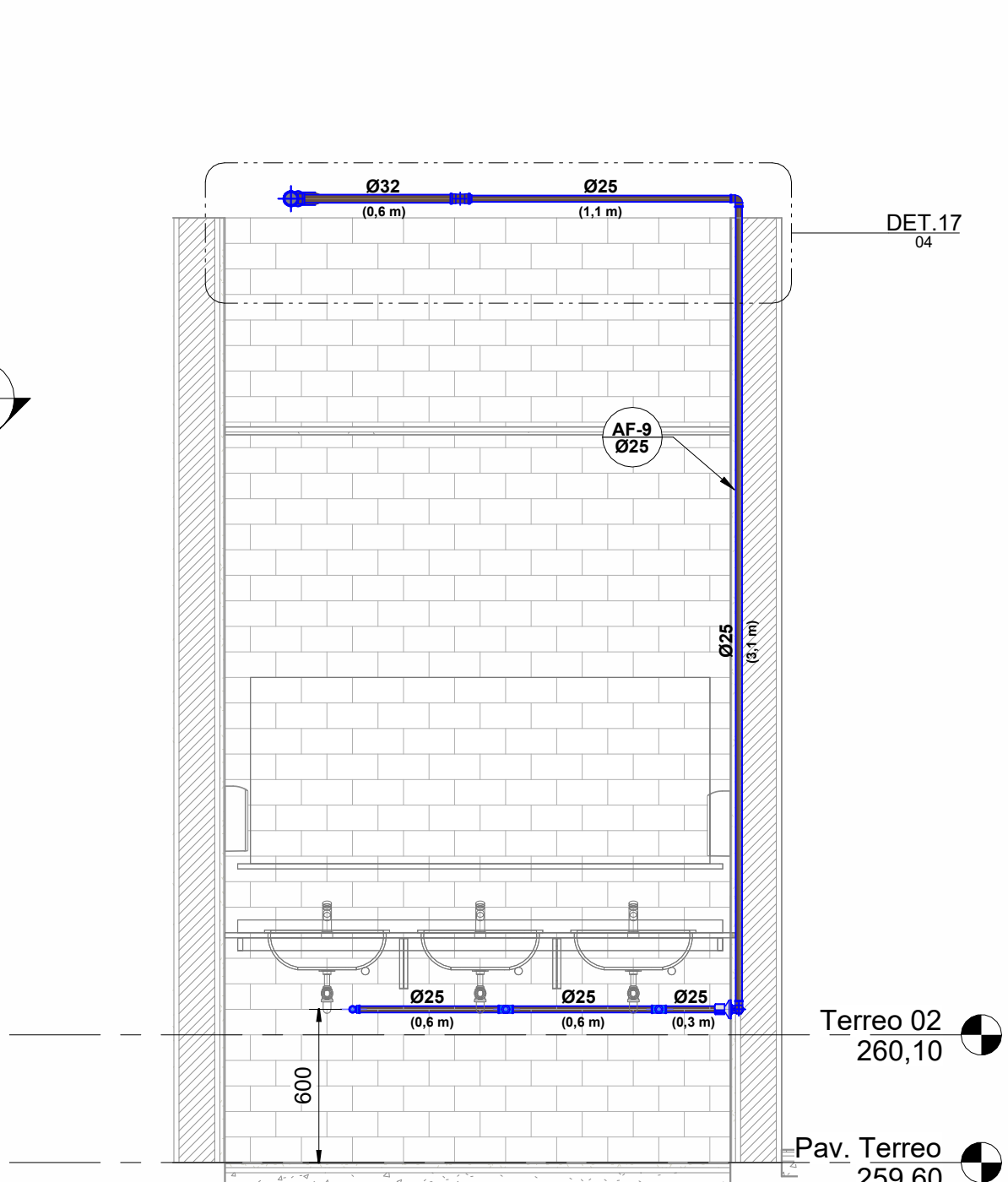
DET.H3 1 : 25
