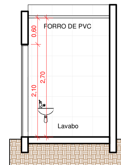
3 CORTE BB ESCALA 1 : 50
