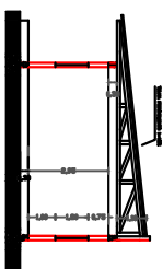
CORTE EF ESC 1:100
