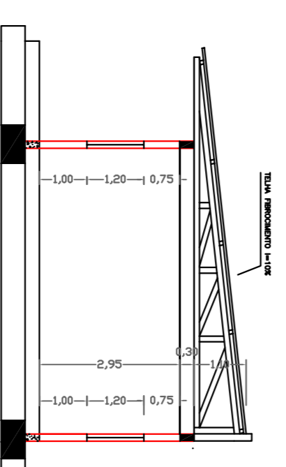
CORTE IJ ESC 1:100
