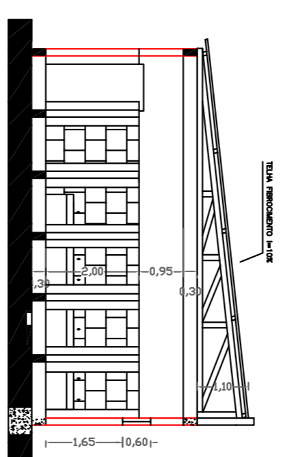
CORTE GH ESC 1:100
