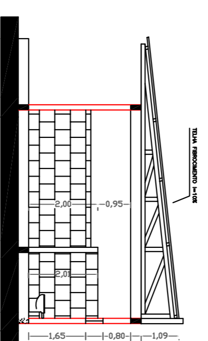
CORTE KL ESC 1:100
