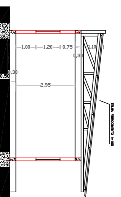
CORTE AB ESC 1:100
