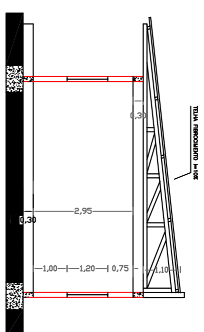
CORTE EF ESC 1:100
