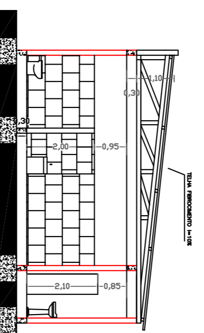
CORTE CD ESC 1:100
